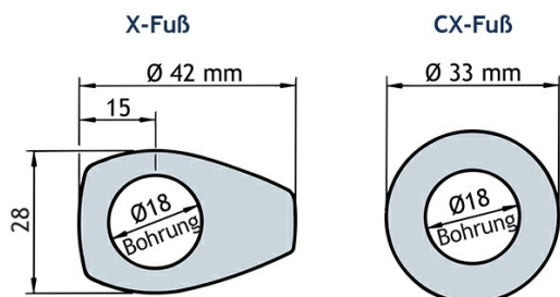
Einbautiefe: 11 mm
