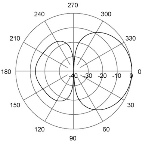
E-Plane | 400 MHz
