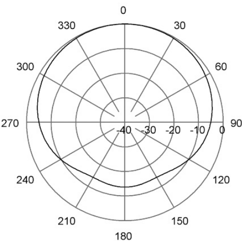
H-Plane | 400 MHz
