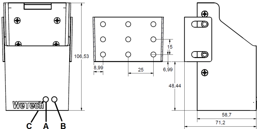
Schemazeichnung WTC642
