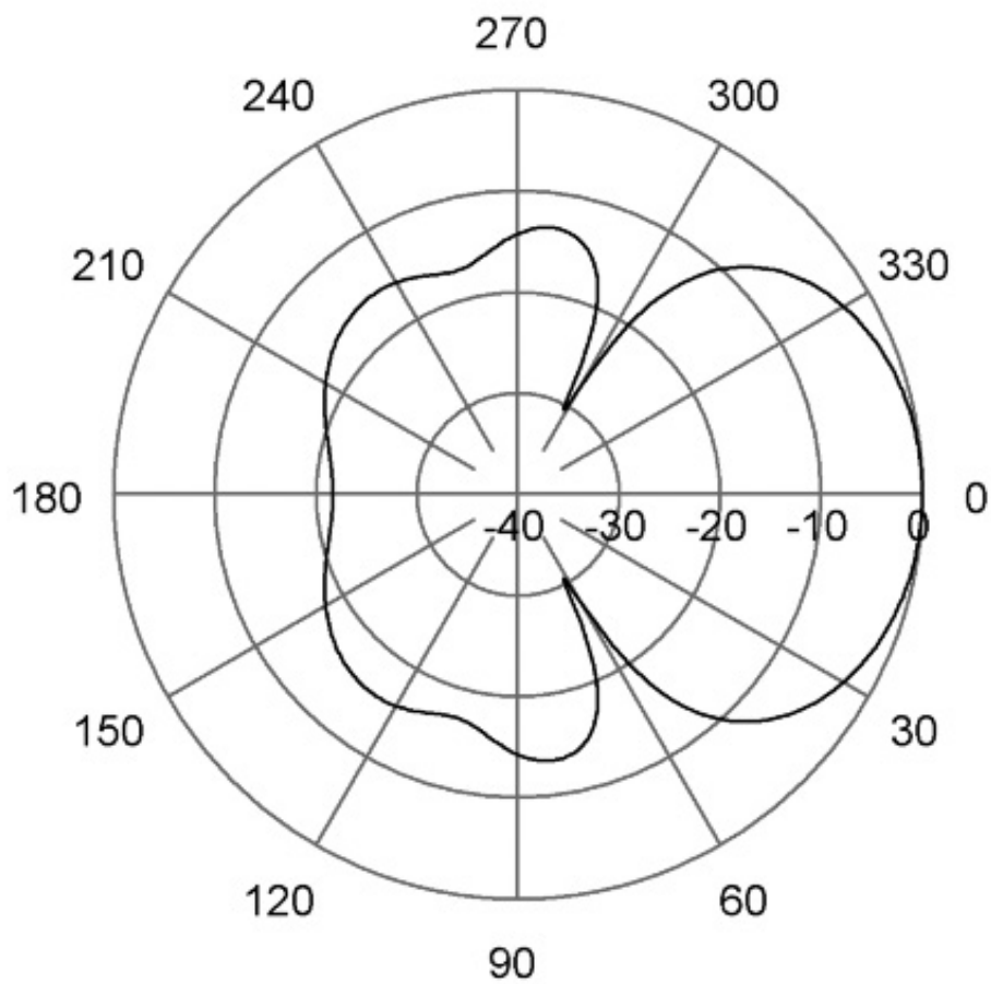
H-Plane | 148 MHz
