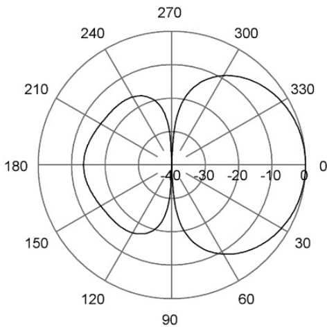
E-Plane | 445 MHz
