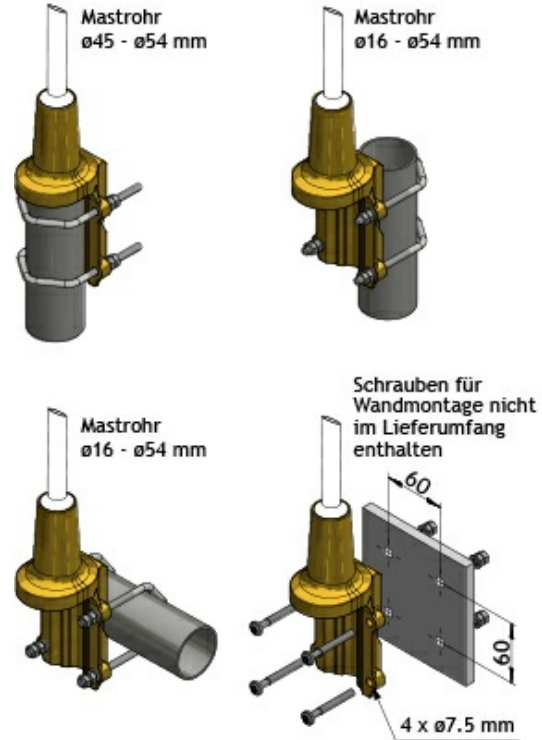
UNIVERSAL-MONTAGEBESCHLAG
