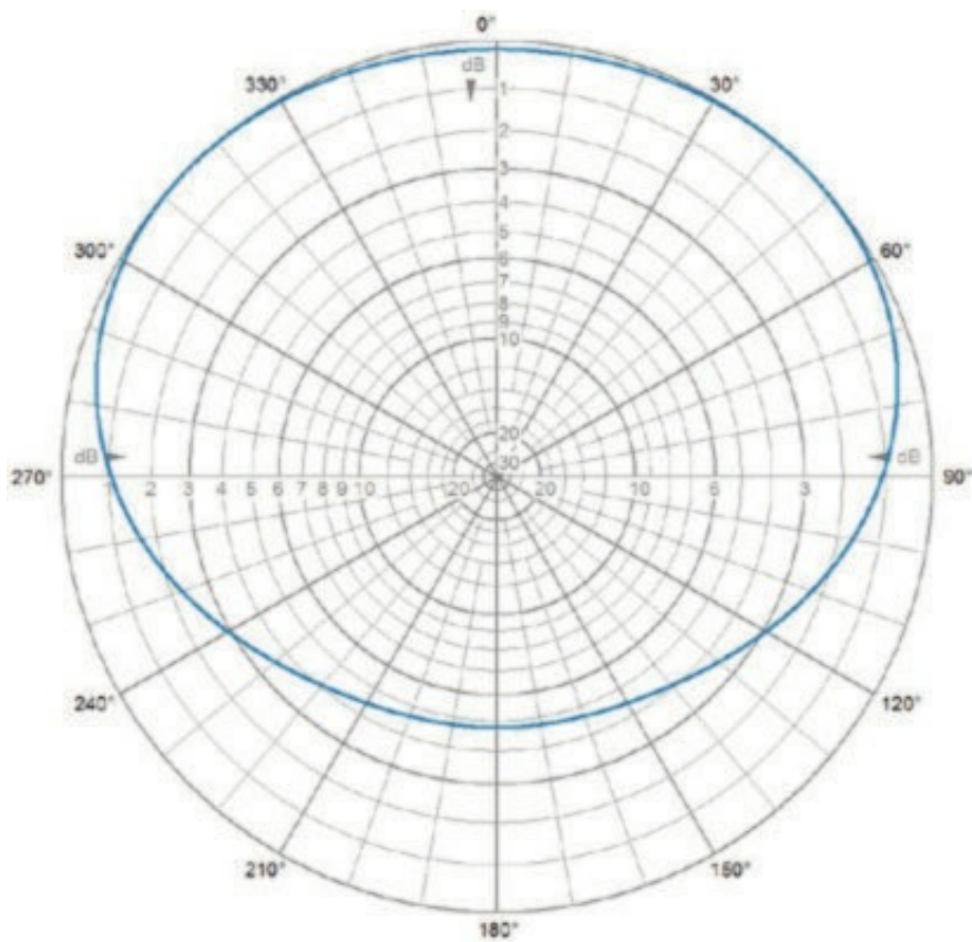
H-Plane | 445 MHz
