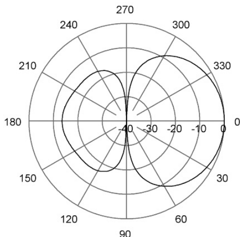
E-Plane | 445 MHz
