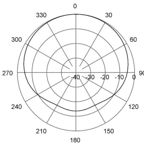
H-Plane | 445 MHz
