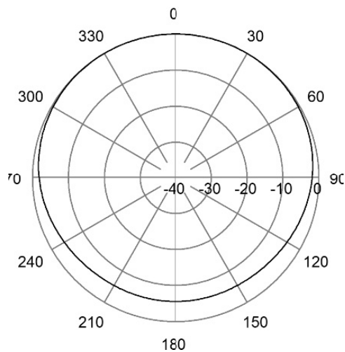
H-Plane | 68 MHz
