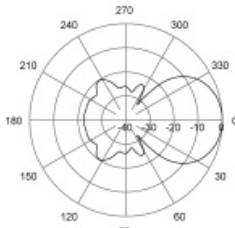
E-Plane | 165 MHz
