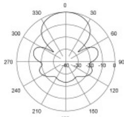
H-Plane | 165 MHz
