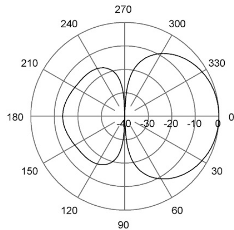
E-Plane | 410 MHz
