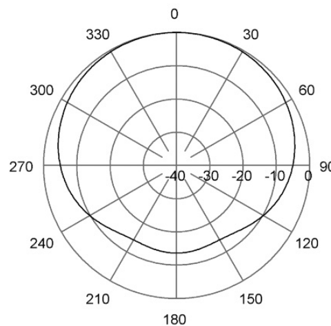
H-Plane | 410 MHz
